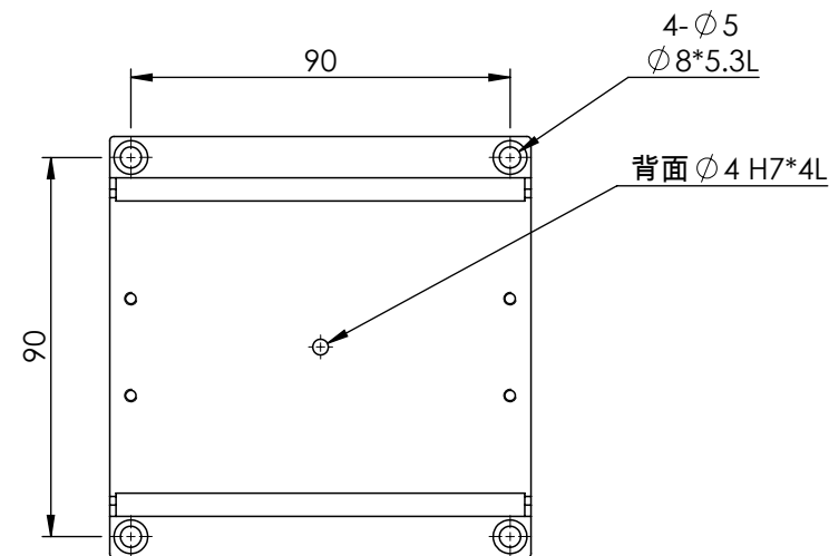
底部安裝孔尺寸
