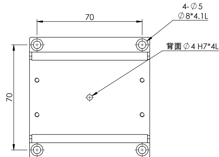
MX(Y)80-S-系列 底座安裝孔尺寸
