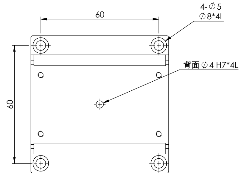
MX(Y)70-S-系列 底座安裝孔尺寸
