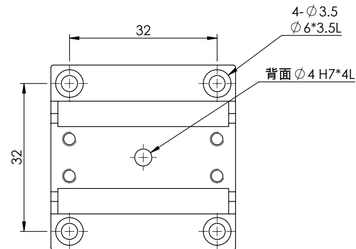
MX(Y)40-S-系列 底座安裝孔尺寸
