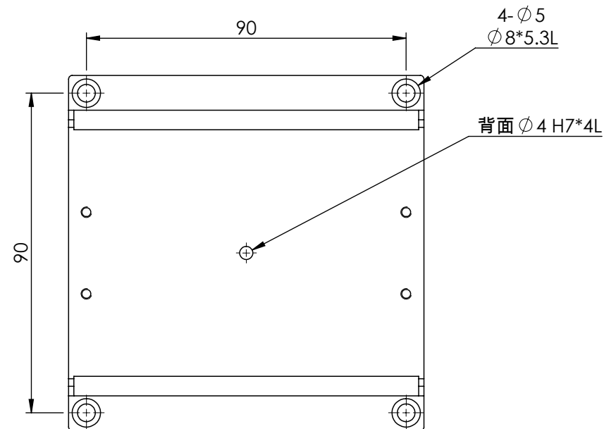
MX(Y)100-S-系列 底座安裝孔尺寸
