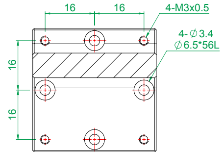
剖面圖 A-A
