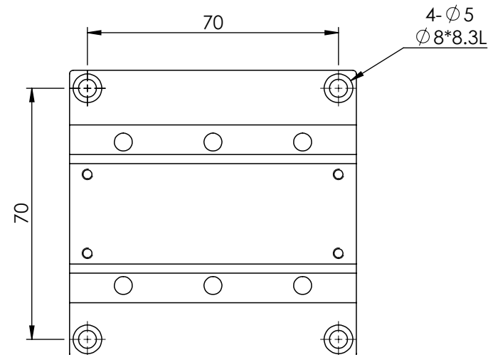
底部安裝孔尺寸
