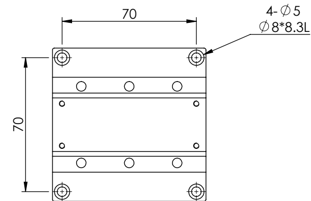
底部安裝孔尺寸
