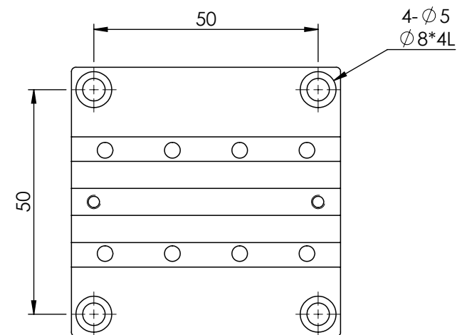
底部安裝孔尺寸
