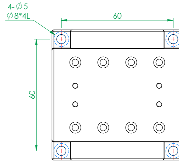
MX(Y)70-A系列 底座安裝孔尺寸
