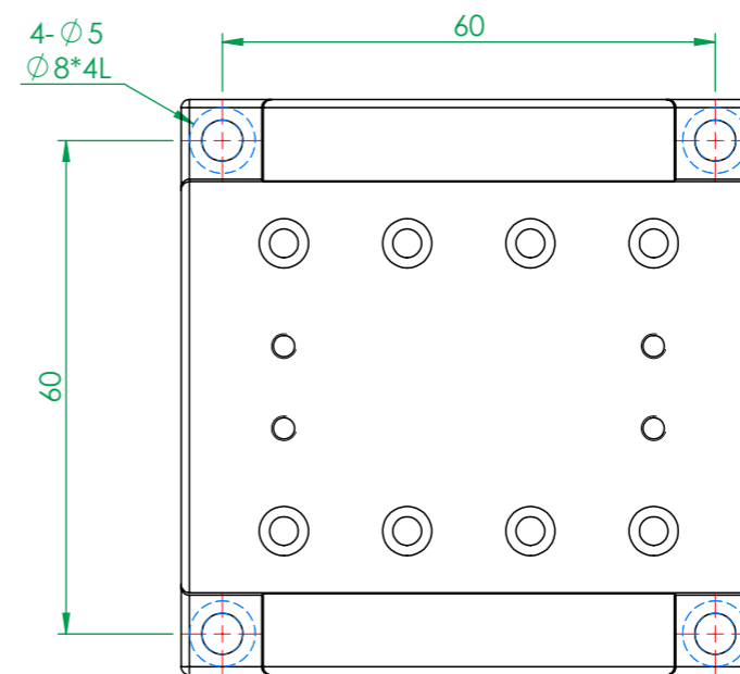
MX(Y)70-A系列 底座安裝孔尺寸
