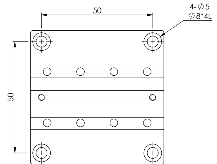
MX(Y)60-A系列 底座安裝孔尺寸
