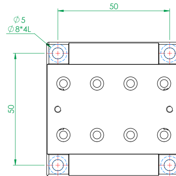
MX(Y)60-A系列 底座安裝孔尺寸
