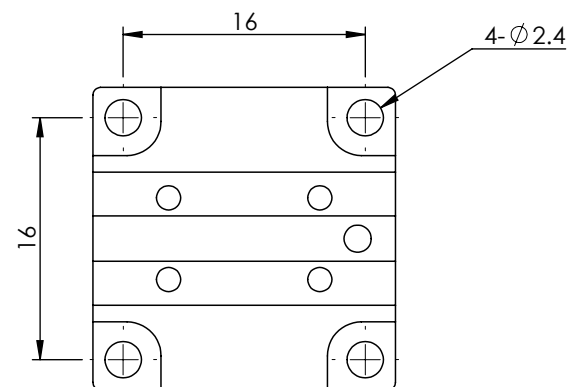
MX-(Y)20-A系列 底座安裝孔尺寸
