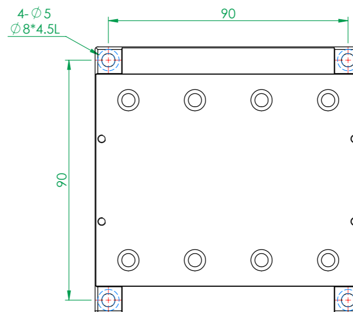
MX(Y)100-A系列 底座安裝孔尺寸
