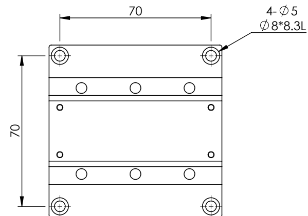
底部安裝孔尺寸
