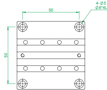
MX(Y)60-A-18系列 底座安裝孔尺寸
