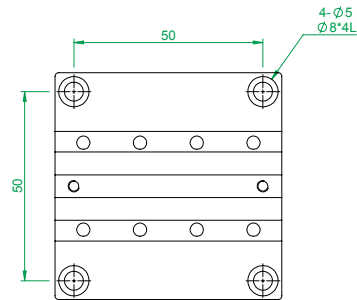
MX(Y)60-A-18系列 底座安裝孔尺寸
