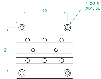
MX(Y)50-A-18系列 底座安裝孔尺寸
