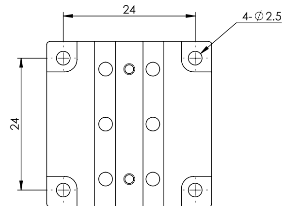
底部安裝孔尺寸
