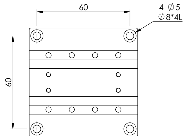
MX(Y)70-A-18系列 底座安裝孔尺寸
