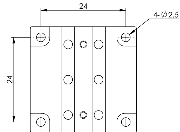
MX(Y)30-A-18系列 底座安裝孔尺寸
