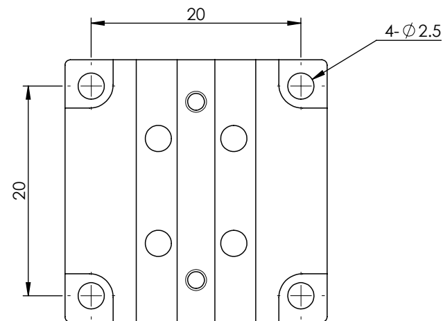
MX(Y)25-A-18系列 底座安裝孔尺寸
