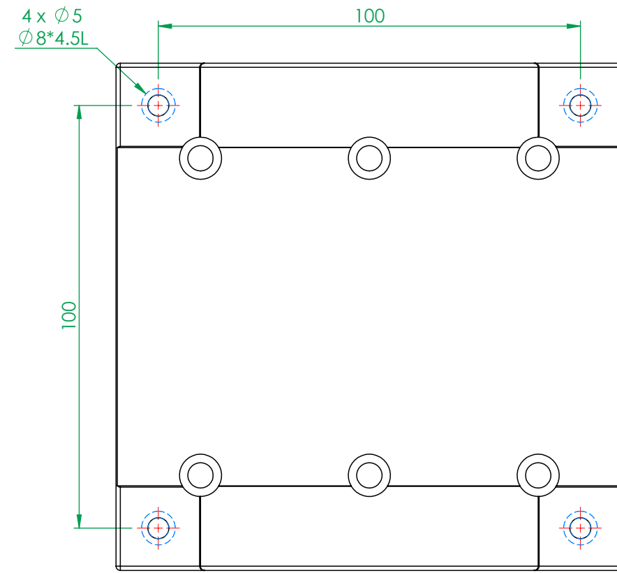
MX(Y)120-A-18系列 底座安裝孔尺寸
