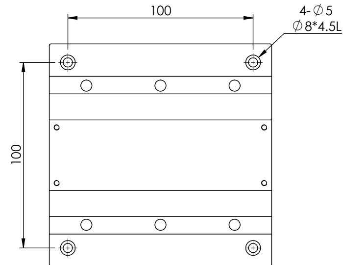
MX(Y)120-A-18系列 底座安裝孔尺寸
