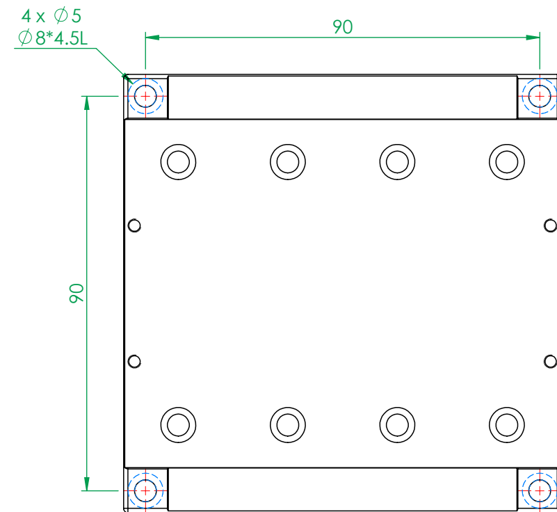
MX(Y)100-A-系列 底座安裝孔尺寸
