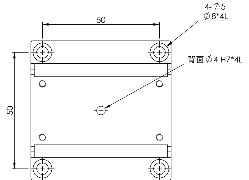
底部安裝孔尺寸
