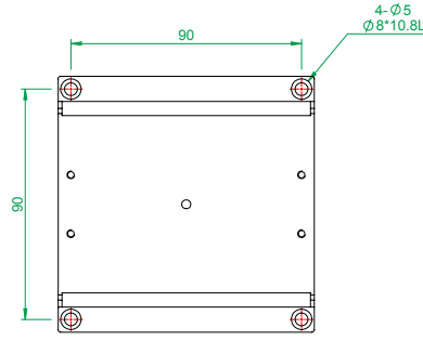
MX(Y)100-S-28系列 底座安裝孔尺寸
