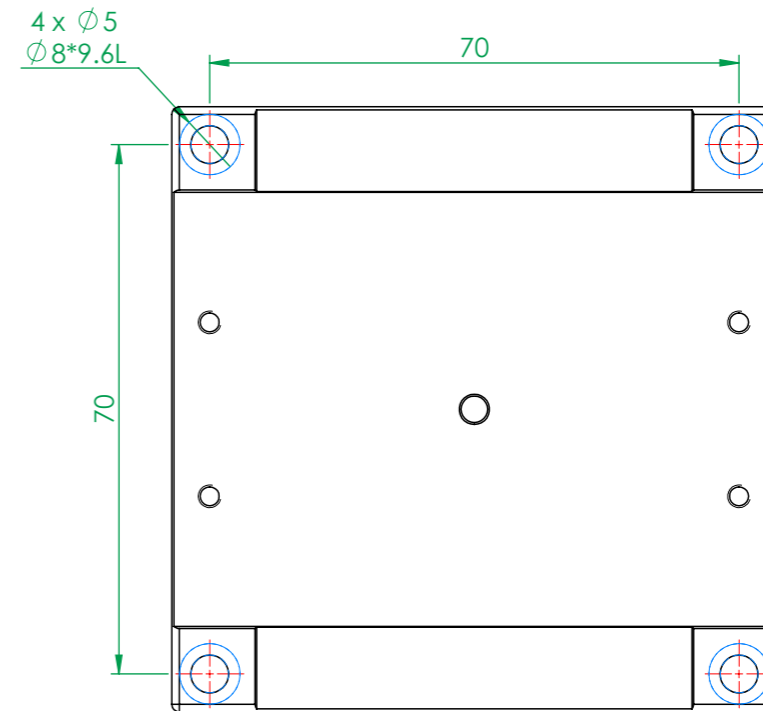
MX(Y)80-S-28系列 底座安裝孔尺寸
