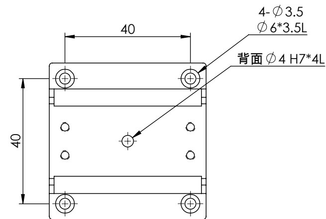
MX(Y)50-S-28系列 底座安裝孔尺寸
