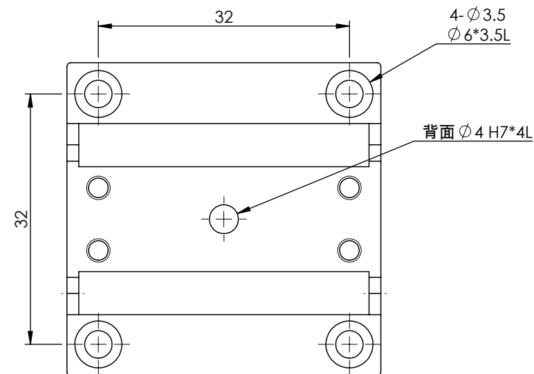
MX(Y)40-S-28系列 底座安裝孔尺寸
