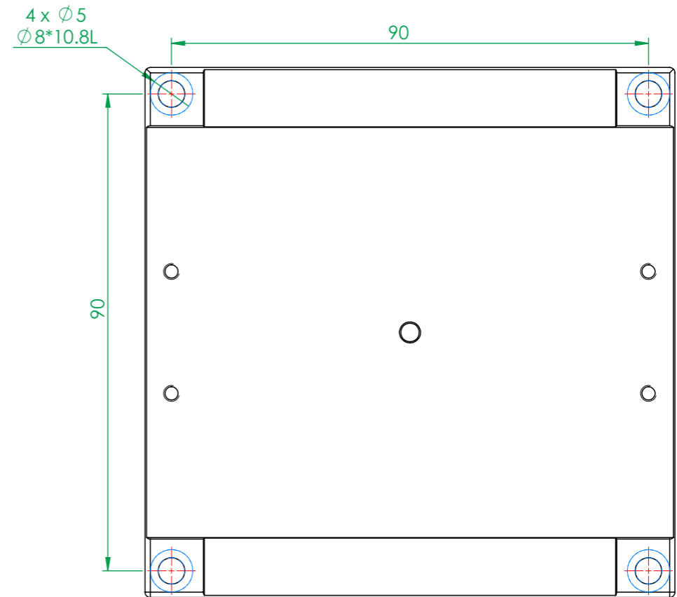
MX(Y)100-S-28系列 底座安裝孔尺寸
