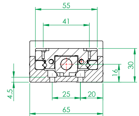
剖面圖 K-K
