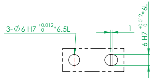
細部放大圖 H 比例 2:2.5
