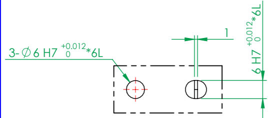
細部放大圖 H 比例 2:2.5
