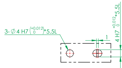
細部放大圖 H 比例 1:1
