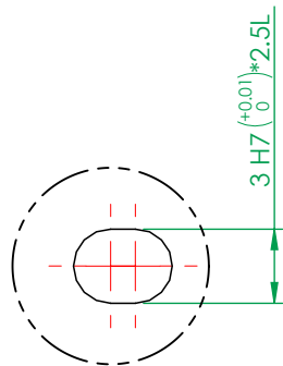
細部放大圖 H 比例 3:1
